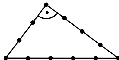
Thalessatz
