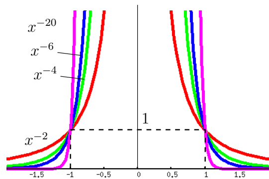
n < 0 gerade
