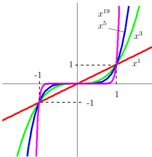
n > 0 ungerade
