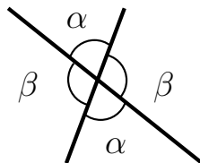
Scheitelwinkel
