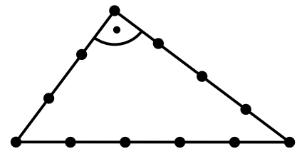
Thalessatz
