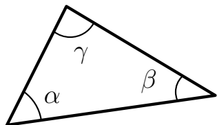
Winkelsumme
