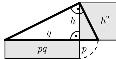
Höhensatz
