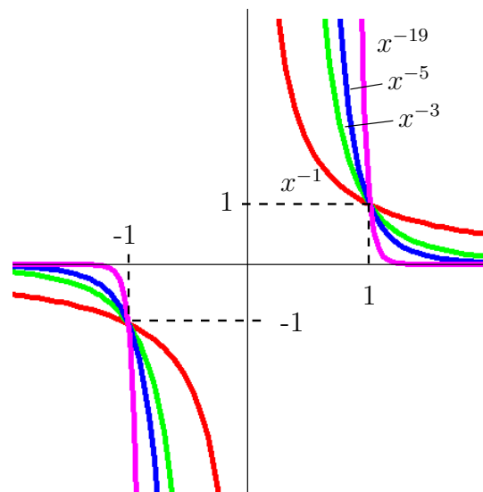
n < 0 ungerade
