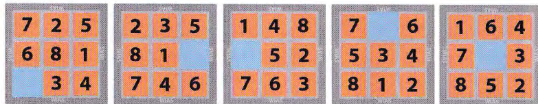
Abbildung 4: Welche dieser Rätsel lassen sich in Abbildung 2, welche lassen sich in Abbildung 3 überführen?
